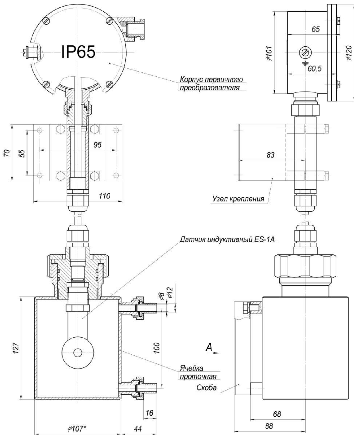
Рисунок А.4 - Габаритные и монтажные размеры анализатора в корпусе «Н» с узлом крепления и проточной арматурой (с индуктивным сенсором ES3-1A)
