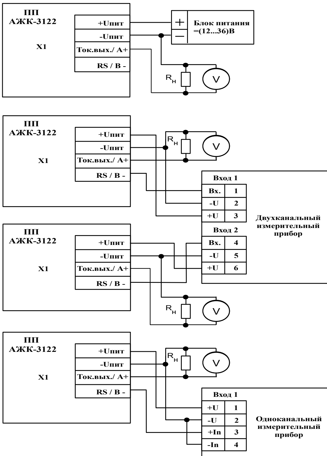
Рисунок С.1 - Схема внешних соединений анализаторов с выходным унифицированным сигналом постоянного тока
