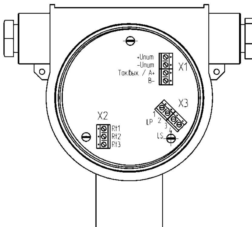
Рисунок В.2 - Вид со стороны задней панели (корпус «И»)
